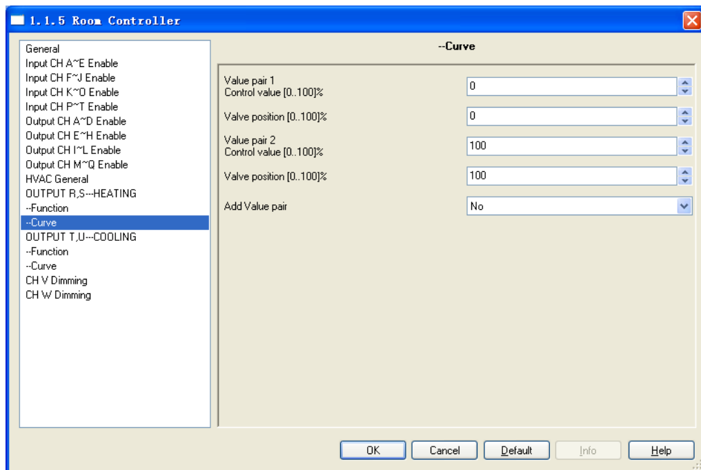
Fig. 5.37 parameter window “HEATING: Curve”
