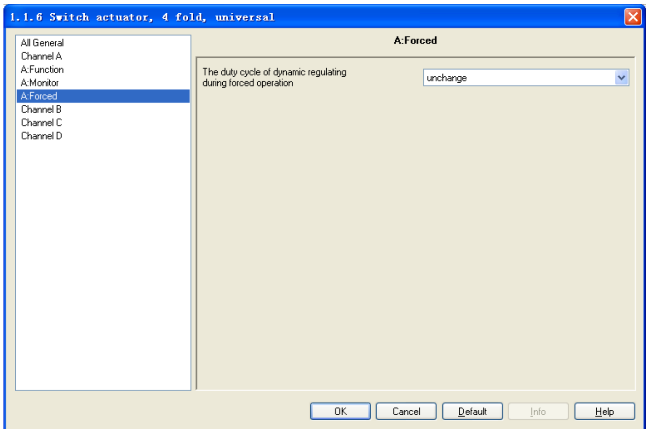
Fig. 2.18 parameter window “X: Forced”
