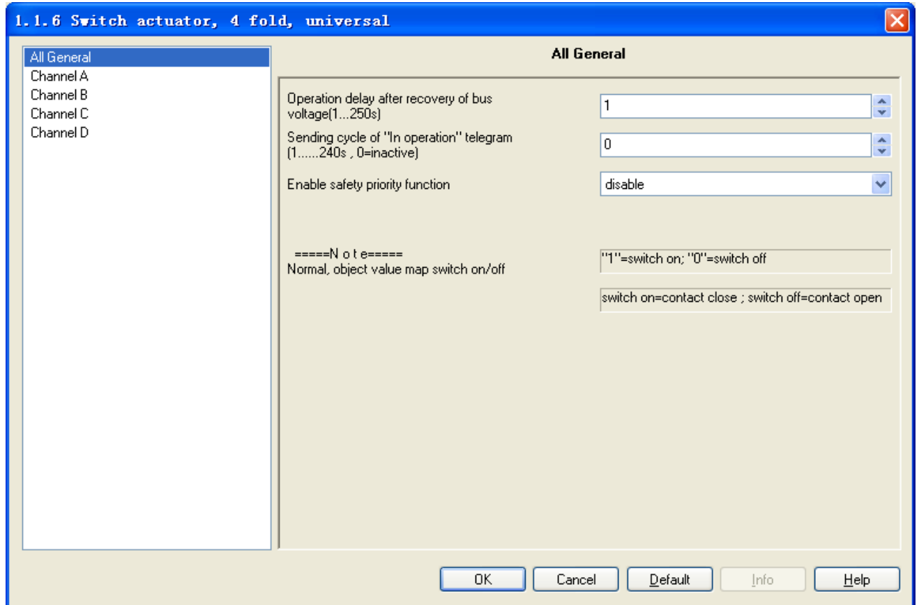
Fig. 2.1 parameter window “All General”
