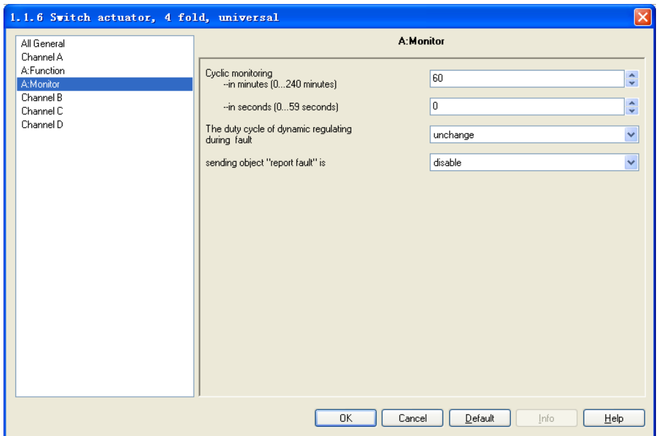
Fig. 2.17 parameter window “X: Monitoring”
