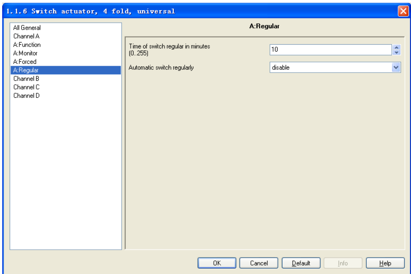
Fig. 2.19 parameter window “X: Regular”
